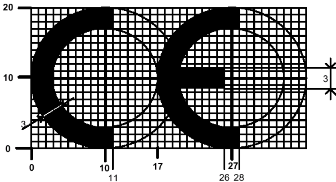
Şekil-1 CE işaretinin ölçüleri
